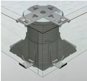
Bei einer Stufencke müssen zwei Clips verlegt werden.
