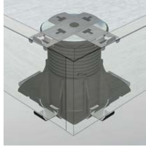
Bei einer Stufenecke müssen zwei Clips verlegt werden.
